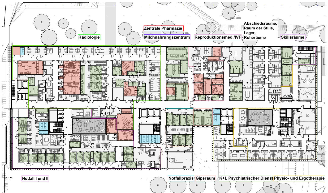
Grundriss Erdgeschoss
